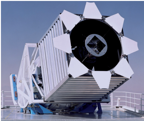
Das 2.5-m-Teleskop des Sloan Digital Sky Survey
